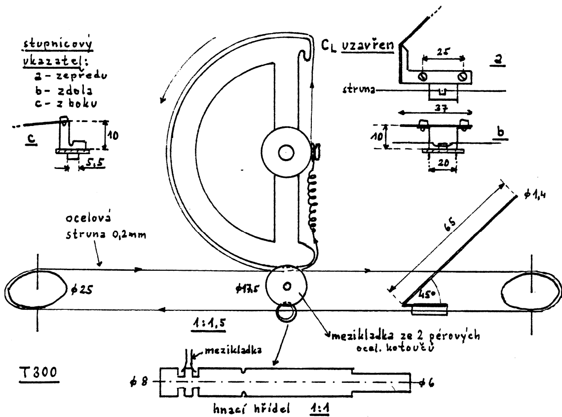
Obr. 5. Stupnicové převody a stupnicový ukazatel.
