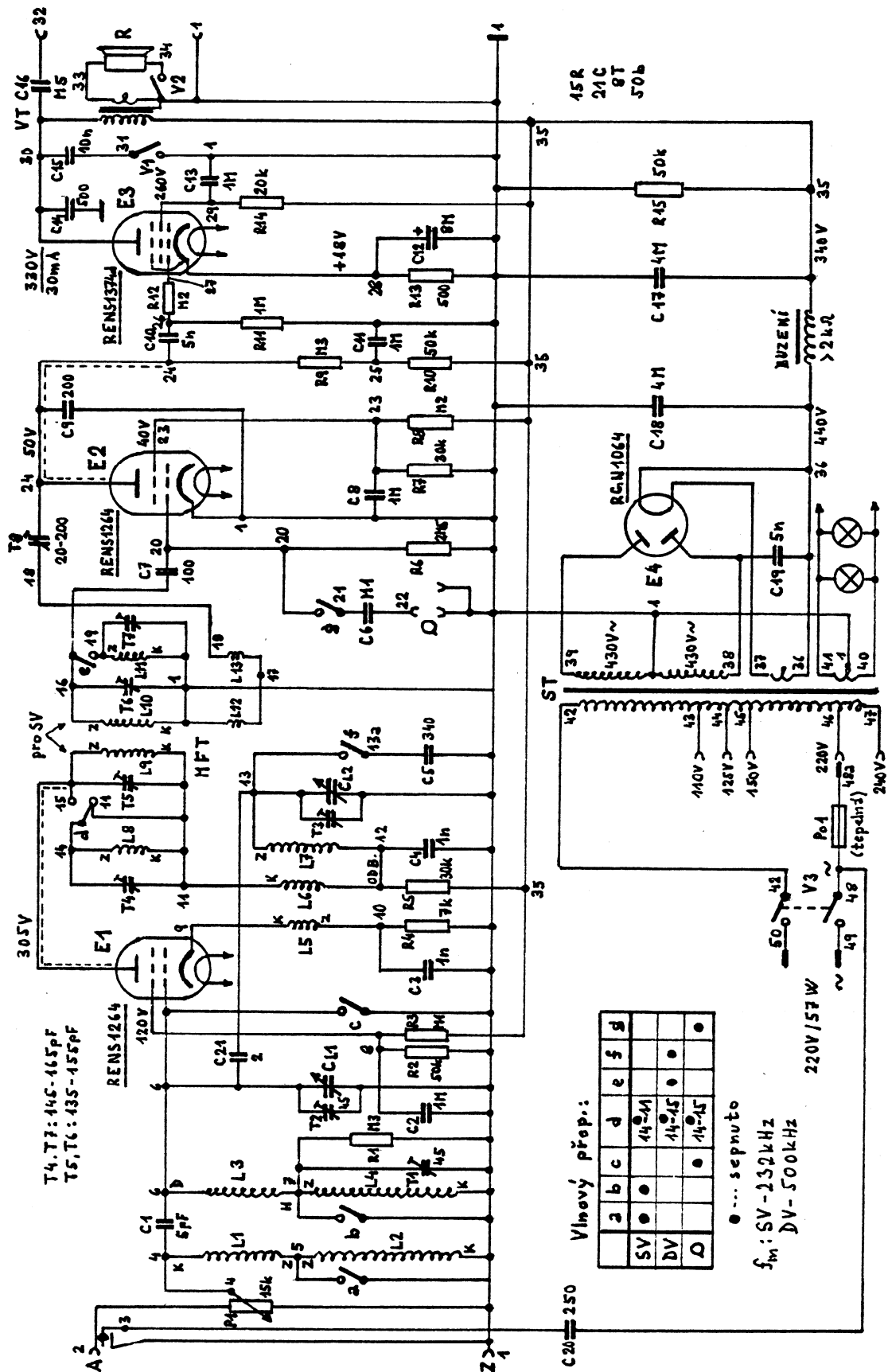
Obr. 1. Schéma zapojení přístroje Telefunken 300.
